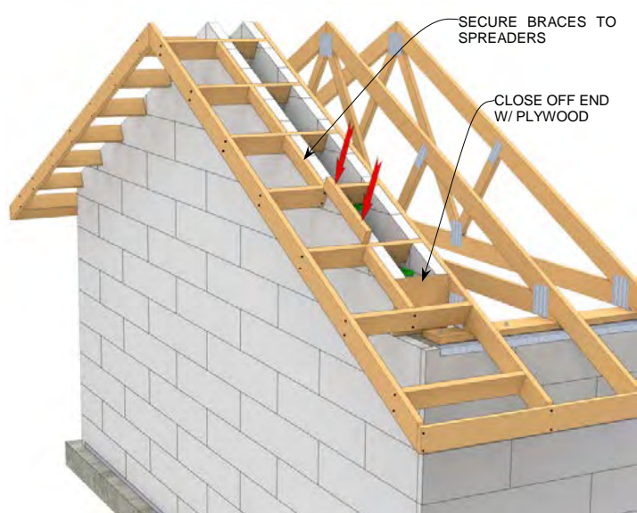
STEP 4 Securing Top Foam - Ready for Pour
